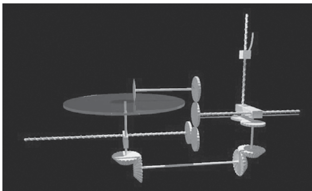
Mecanismo de un carro transportador diseñado por Daniel Yule, del Movimiento de Juventudes Larouchistas. La animación puede verse en http://tinyurl.com/37qv51 .
