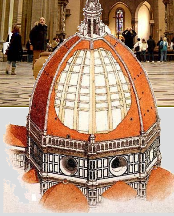
Filippo Brunelleschi introdujo el principio físico de la catenaria en la construcción de la gran cúpula de la catedral de Florencia. El corte transversal en la cúpula muestra la estructura interna. (Fotos: Ricardo André Frantz [izq.]; cortesía de Pennie Sabel).
