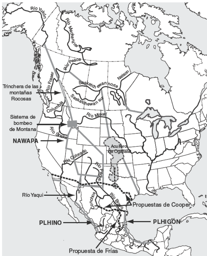
Esquema conceptual de la Alianza Hidráulica y Energética de Norteamérica, NAWAPA, para llevar agua de Alaska, donde abunda, al oeste de Estados Unidos y el norte de México, donde escasea. (Fuentes: Parsons Company, Manuel Frías Alcaraz, EIR).
