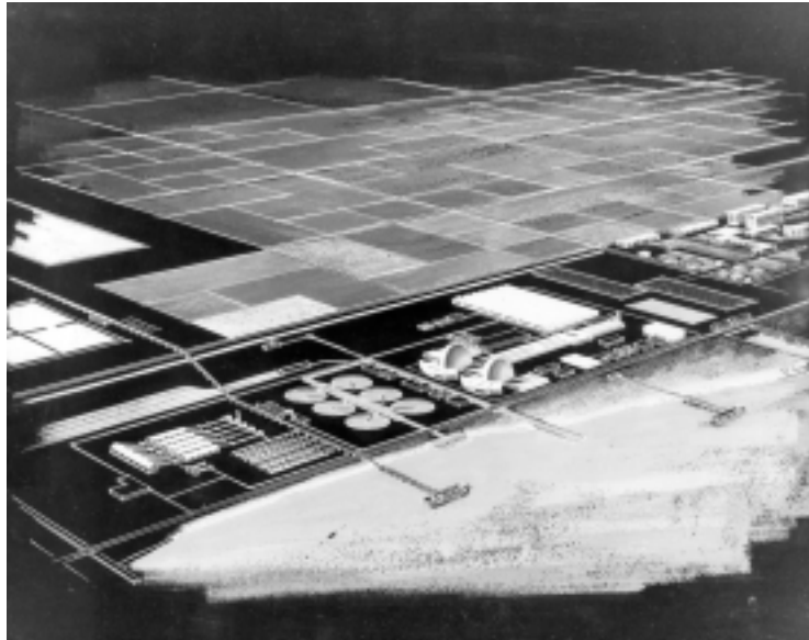
Complejo nuclear agroindustrial. En este diseño de 1969, dos reactores nucleares generarían más de 2.000 megavatios de electricidad y hasta mil millones de galones diarios de agua dulce desalando agua de mar. Enseguida se aprecia un centro agroindustrial de 300.000 acres, con la capacidad de alimentar a 6 millones de personas. La central alimenta de energía a todas las instalaciones, y a las zonas residenciales de la derecha. (Ilustración: Comisión de Energía Atómica de EU).
